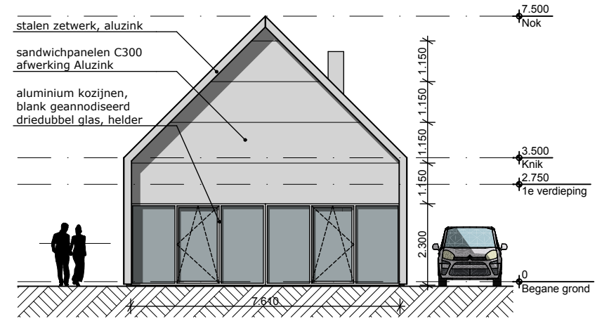
Kopgevel 1 (vide)
