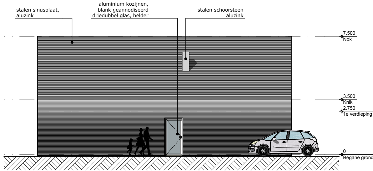
Zijgevel 1
