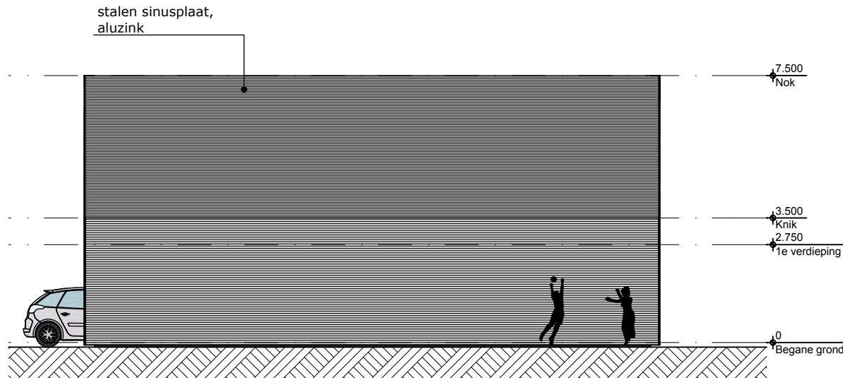
Zijgevel 1
