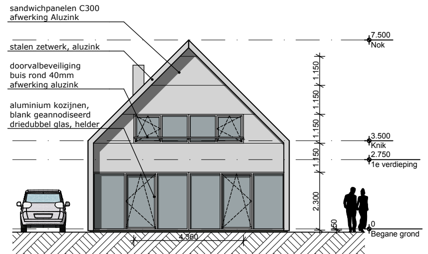
Kopgevel 1 (vide)
